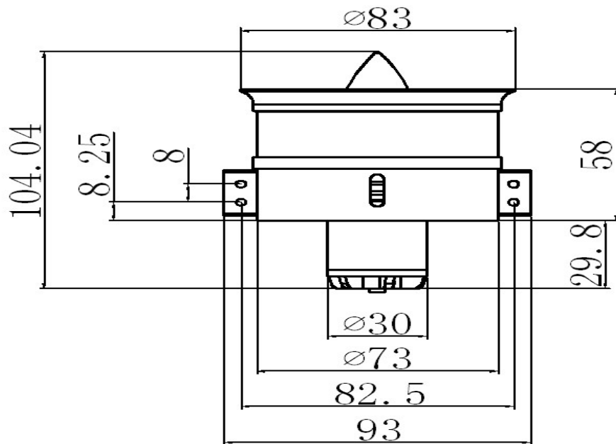
尺寸图 dimensional drawing(mm)
